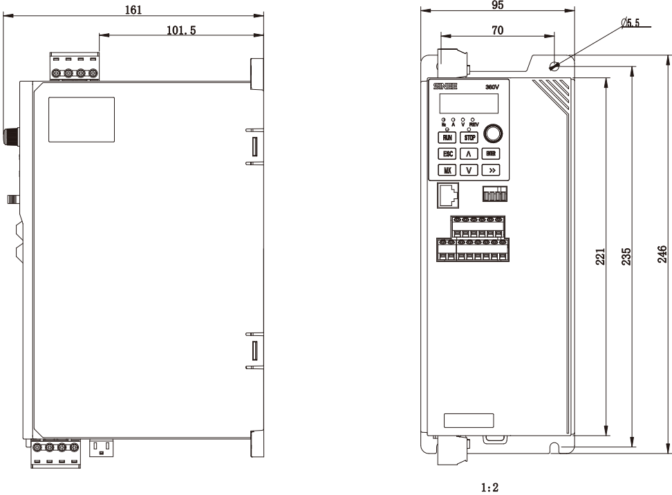
(c) E700-5R5-3B-G Size
